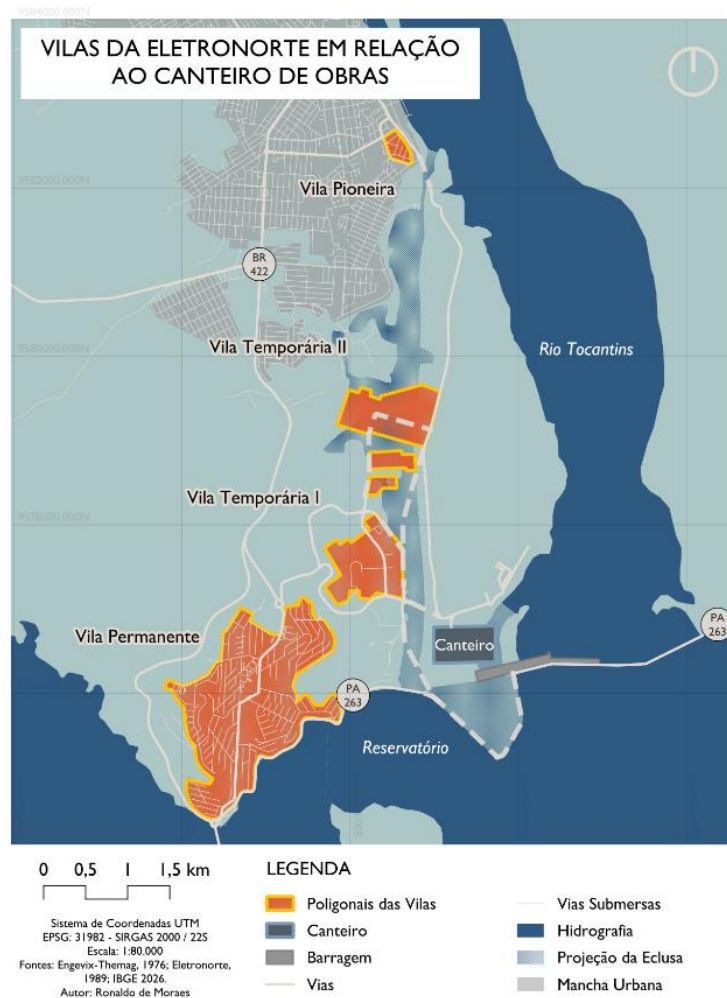
Figura 5 – Vilas da Eletronorte em relação ao canteiro da UHE-Tucuruí.
