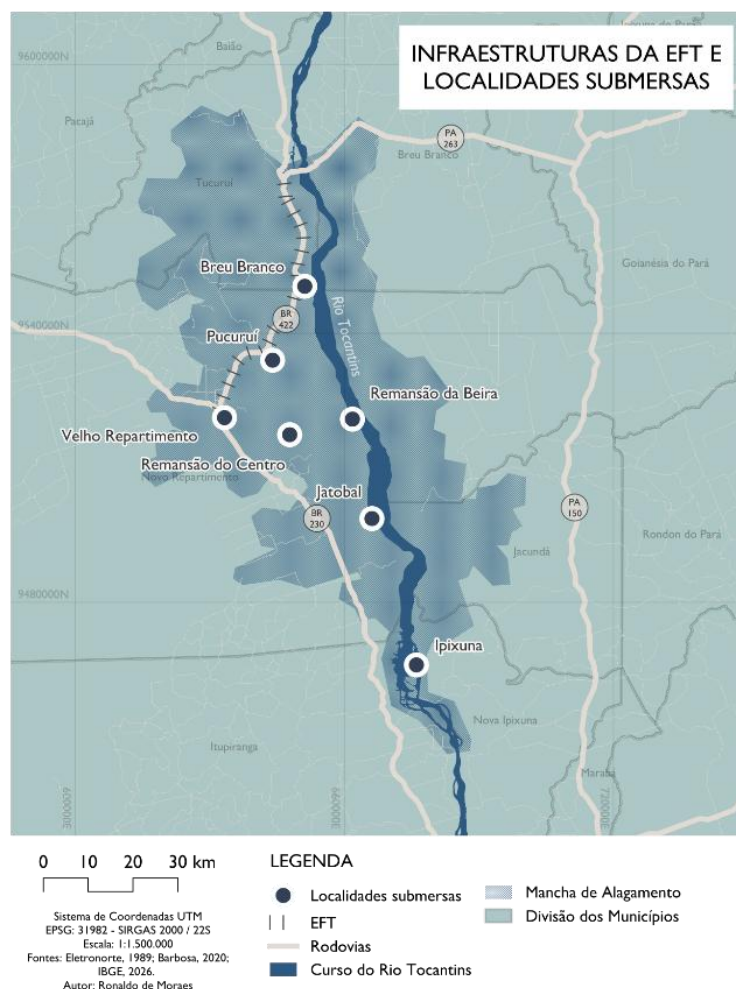
Figura 7 – Núcleos urbanos e trilhos da EFT submersos pelo lago da UHE-Tucuruí.
