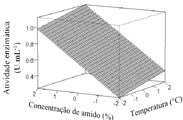
Figura 2 - Superfície de resposta para atividade de amilase conforme variação da concentração de amido e da temperatura.
